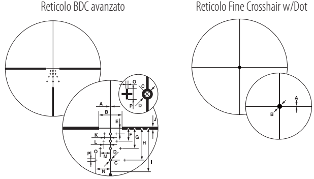
Le lettere da A a P nel grafico sopra fanno riferimento alle coperture bersaglio in funzione del reticolo indicate nella tabella a destra.
