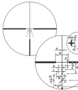
Kompaktes BDC-Fadenkreuz
