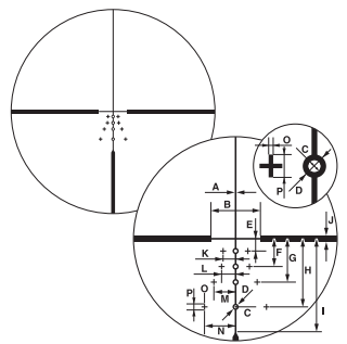
Усовершенствованная визирная сетка BDC
