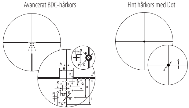
Bokstäverna A till P bilderna ovan refererar till hårkorsets medförstoring med uppgifterna A till P som visas i tabellen till höger.
