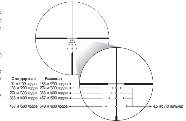
Усовершенствованная визирная сетка BDC
