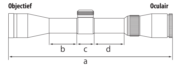
De letters a t/m d in de bovenstaande afbeelding verwijzen naar de lengten (a) t/m (d) in de tabel Specificaties.
