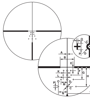
Zaawansowana siatka celownicza BDC
